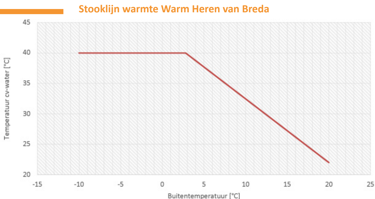
Figuur 3 – Stooklijn warmte
